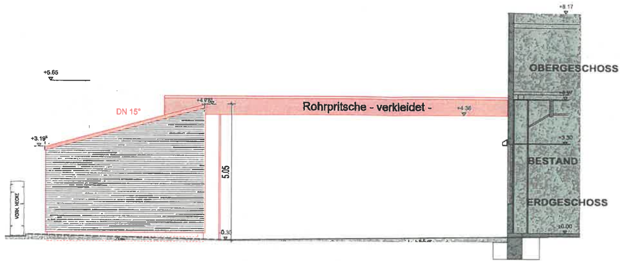
NORDANSICHT
