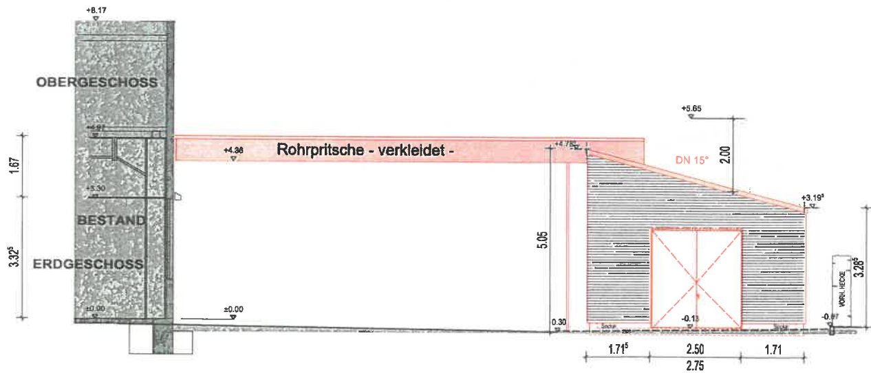
SÜDANSICHT
